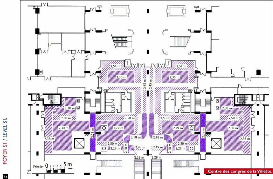
Hauteurs sous plafond - Foyer S1 / Ceiling heights - Level S1
