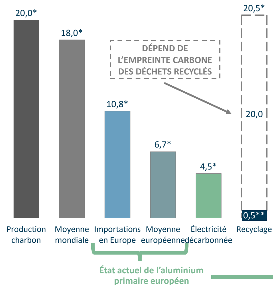
ÉMISSIONS DE CO 2 PAR SOURCE DE PRODUCTION D'ALUMINIUM PRIMAIRE | En tCO 2 / tAl, méthode cradle to gate*
